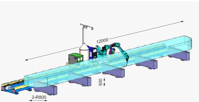
Схема зоны сварки рельсов длиной 12 метров
